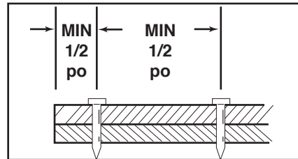
ESPACEMENT – ACIER SUR ACIER
