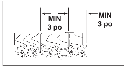
ESPACEMENT – BOIS SUR BÉTON
