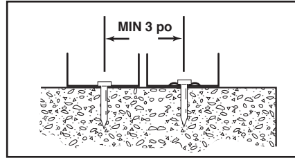
ESPACEMENT – PROFILÉS MINCES SUR BÉTON
