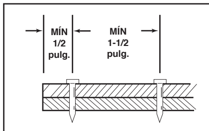
ESPACIO ACERO A ACERO
